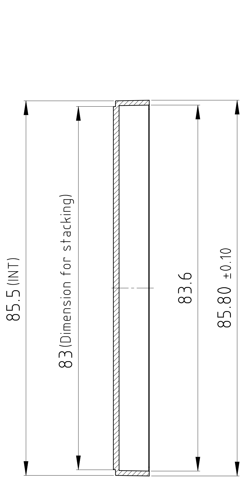
SECTION A-A
