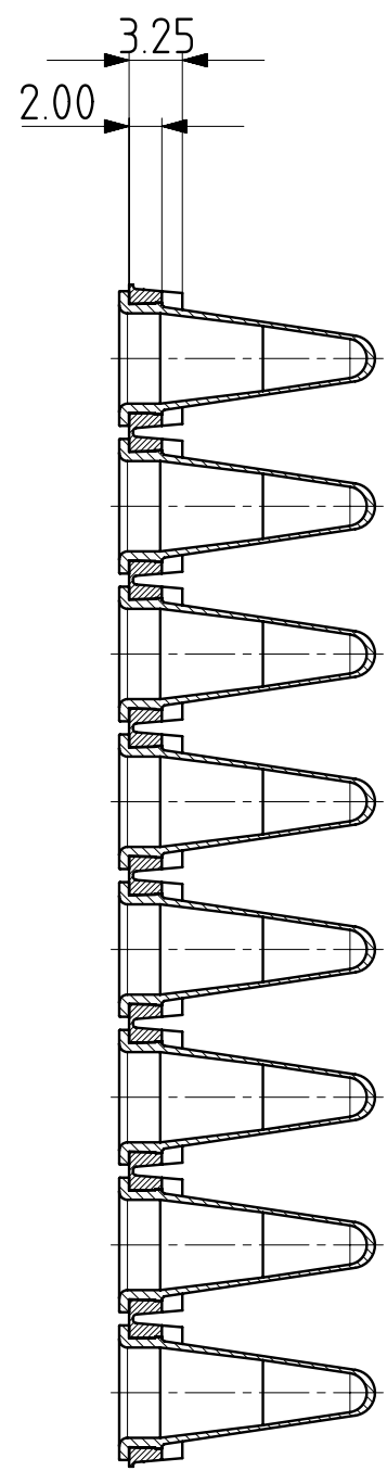
SECTION D-D
